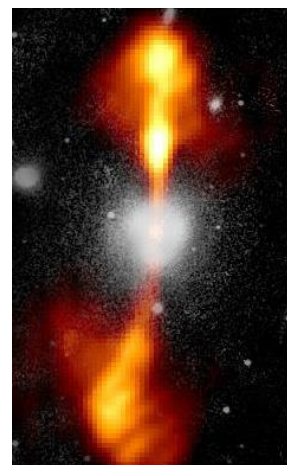
Fig. 15c: La misma galaxia con la imagen de radio superpuesta. Se observan unos chorros de materia coloreados artificialmente de rojo.
