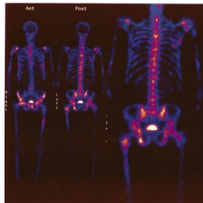
Fig. 20a: Mapa del universo tal como lo ve el "Fermi Gamma-Ray Space Telescope". La línea central es nuestra galaxia. Fig. 20b: Gammagrafía ósea del cuerpo humano
