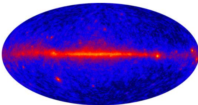
Fig. 20a: Mapa del universo tal como lo ve el "Fermi Gamma-Ray Space Telescope". La línea central es nuestra galaxia. Fig. 20b: Gammagrafía ósea del cuerpo humano
