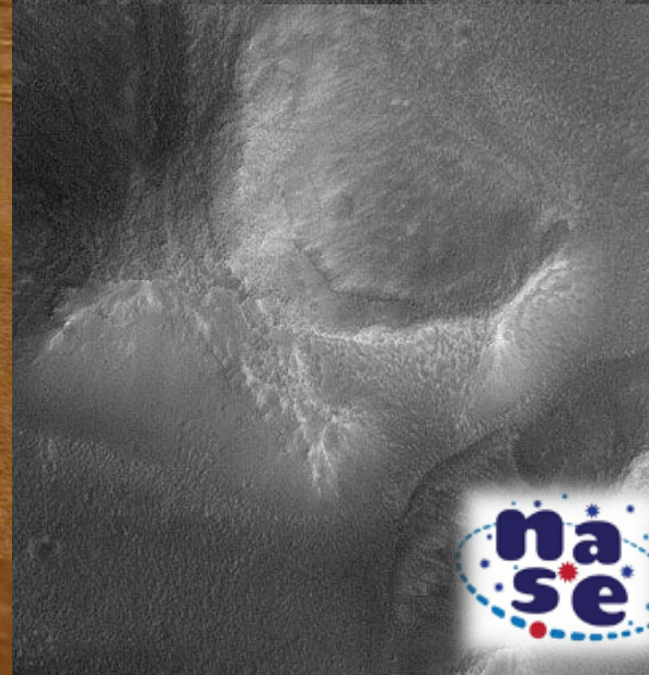
シドニア, 2006年9月, マーズ・エクスプレス
