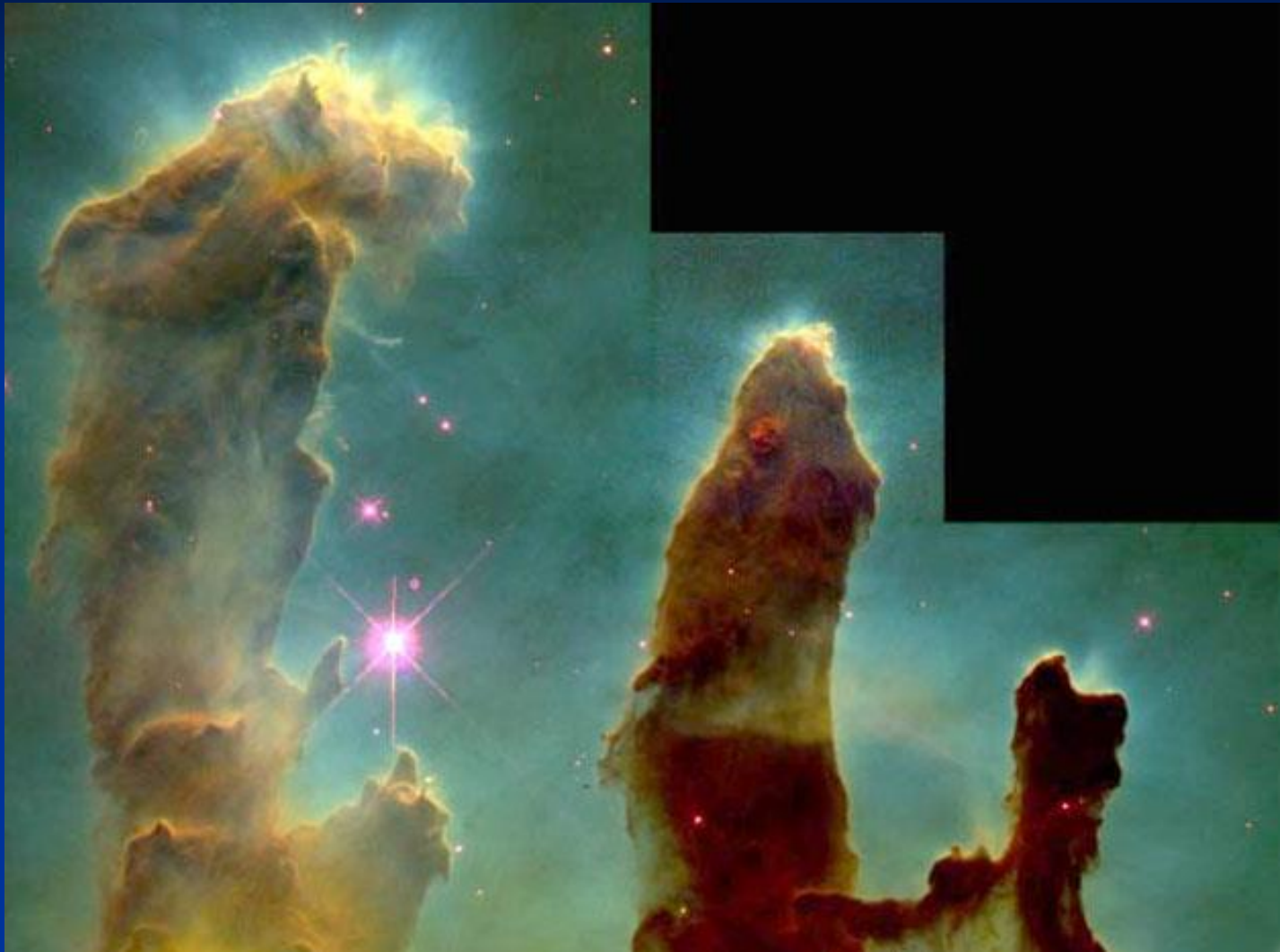
M 16、創世の柱 出典：ハッブル宇宙望遠鏡
