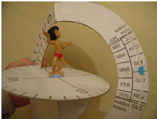
Fig. 30a: Demonstrator pentru latitudinea 70^\circ N, Fig. 30b: latitudinea 20^\circ S.
