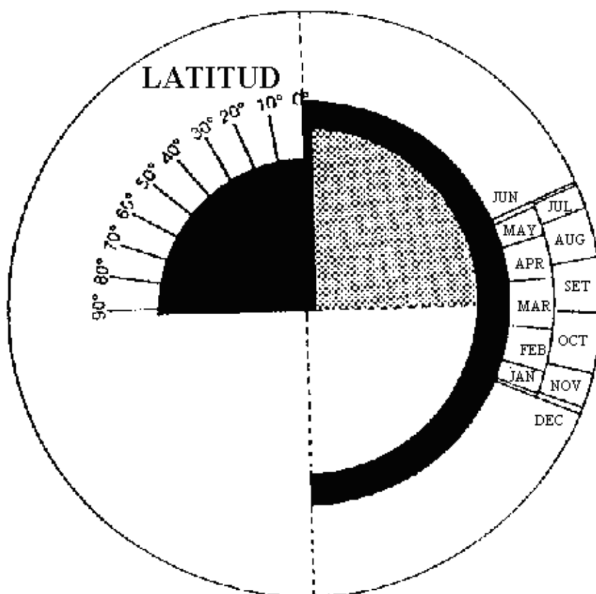
Fig. 12: Piesa principală a unui demonstrator solar pentru emisfera nordică.
