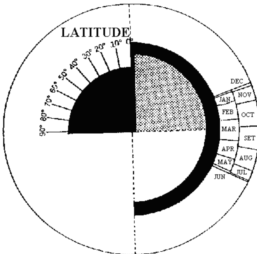
Fig. 14: Componenta principală a unui demonstrator solar pentru emisfera sudică.
