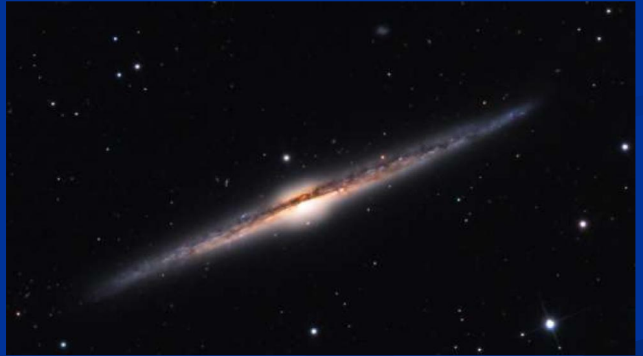
渦巻き銀河エッジオンビュー (クレジットESO=NASA)
