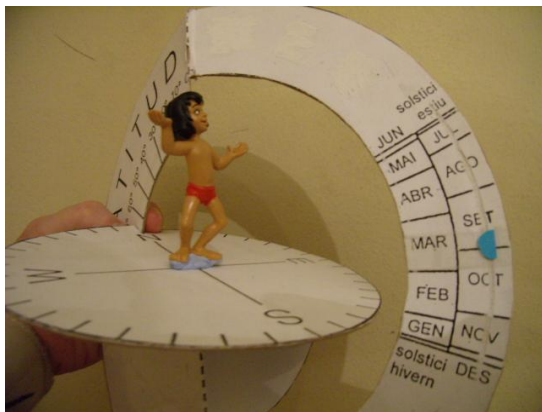
Fig. 38a: Demonstrator for latitude 70° N, Fig. 38b: latitude 20° S.
